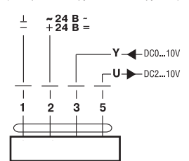
Схема № 4. Аналогове керування 0...10 В (для приводів з пружиною і без пружини)
