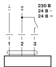
Схема № 2. Двопровідне керування (для приводів без пружини)
