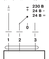
Схема № 3. Однопровідне керування (для приводів з пружиною)
