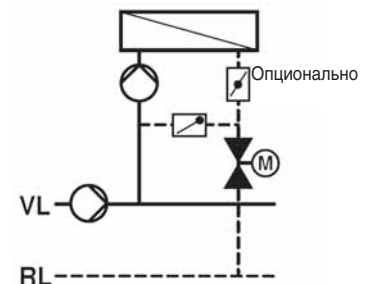
Подмешивание с дросселированием. Применение комбинированного клапана при наличии угрозы замораживания.
