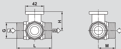
R5... (трехходовой, наружная резьба)
