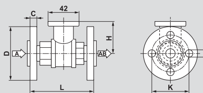
R6... (двухходовой, фланец)
