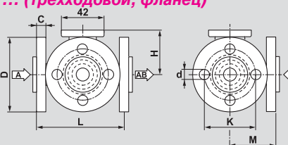
R7... (трехходовой, фланец)
